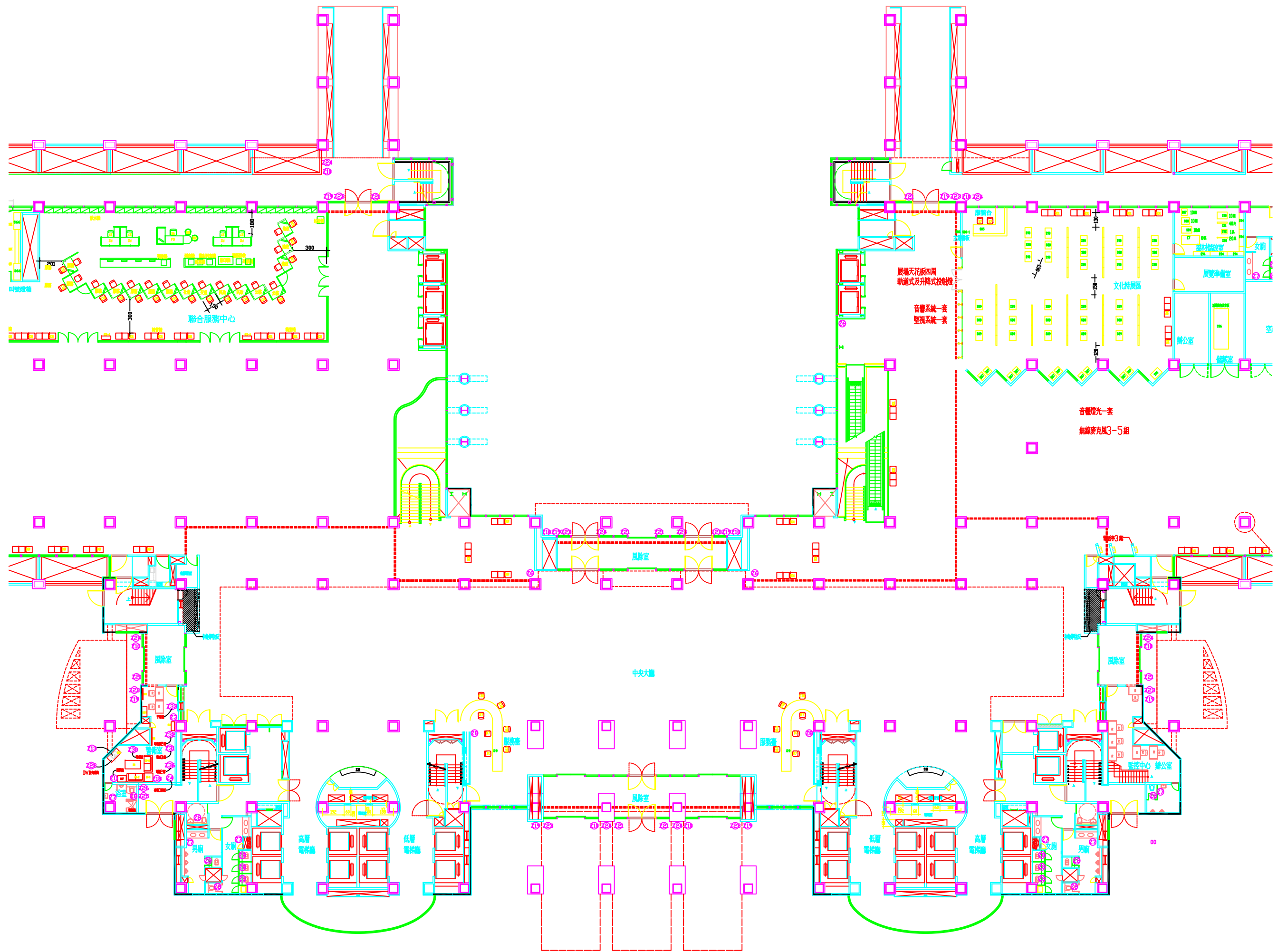
一層平面圖 1/200
